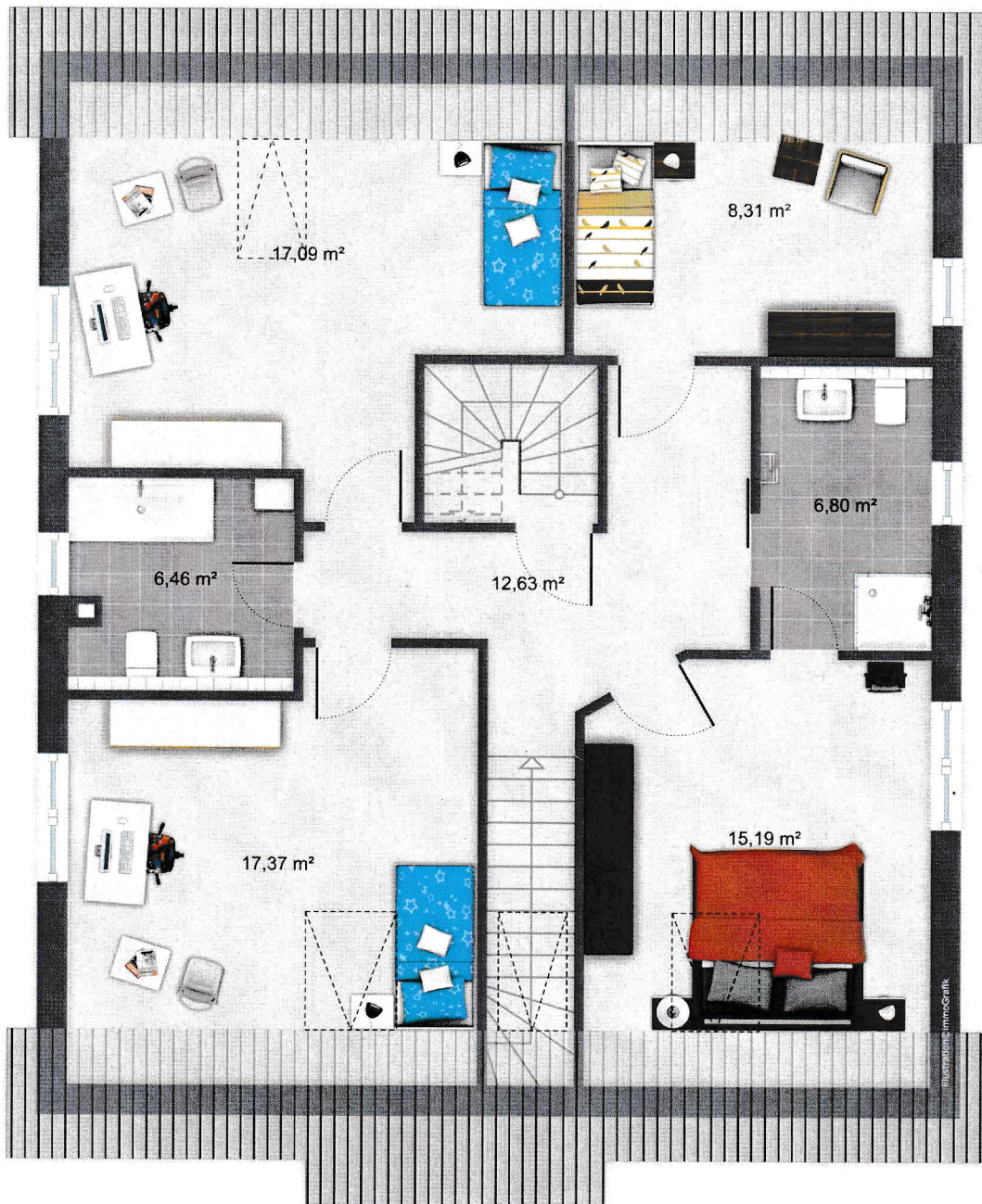
Obergeschoss
